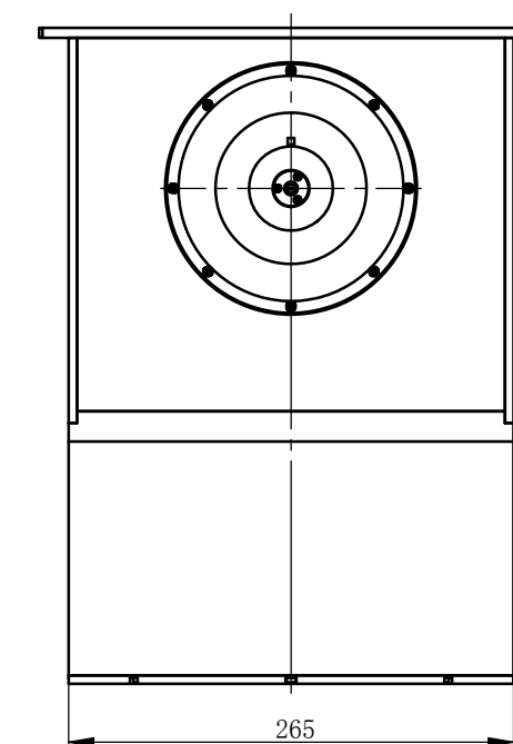
视图 G
